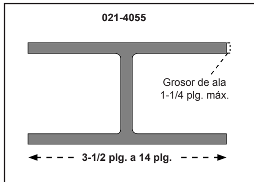
FIGURA 6 - INSTALACIÓN 021-4055
