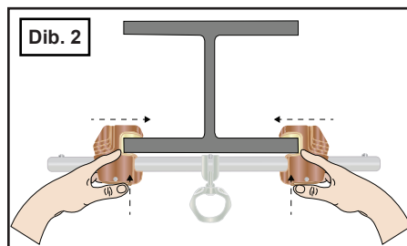
FIGURA 6 - INSTALACIÓN 021-4055
